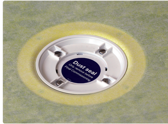
Einbau Ablauf über dem Dichtband
