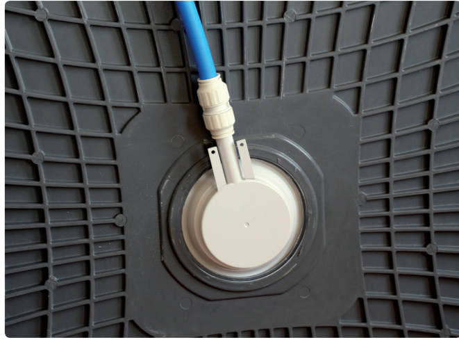
Anbringung Absaug-Ablauf am Duschboard
